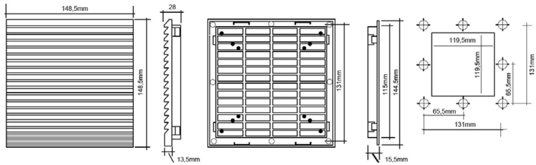
Filtro FK9803
