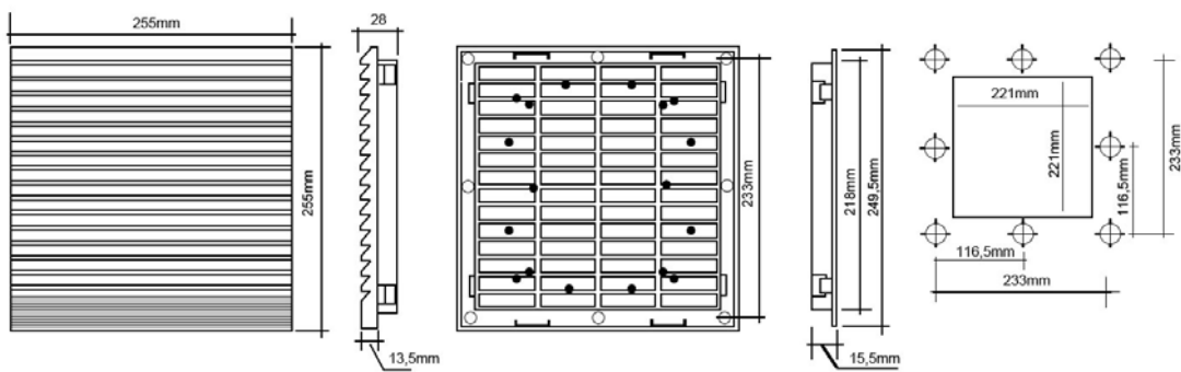
Filtro FB9805
