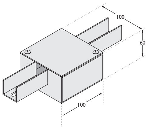
Caixa de Derivação "T"
